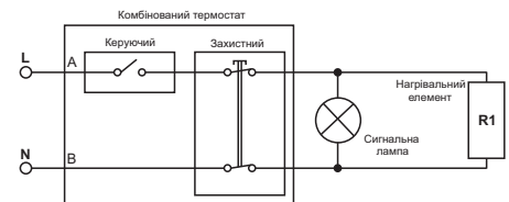
Рис. 6. Схема електрична
